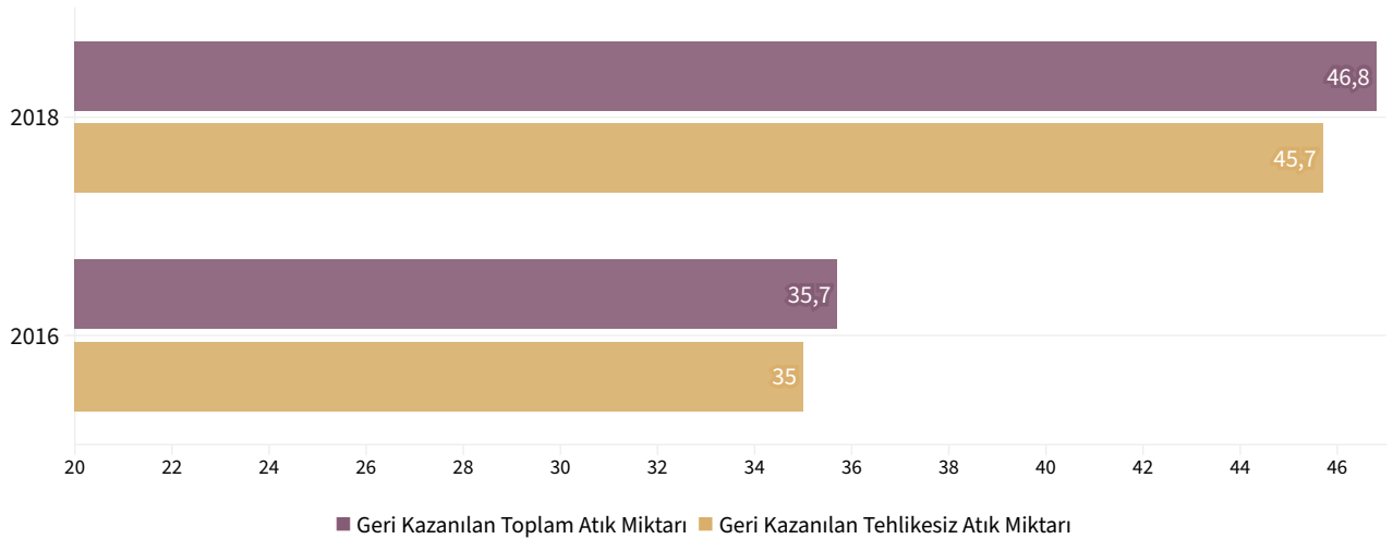
Şekil 175. Yıllara Göre Geri Kazanılan Toplam Atık ve Tehlikesiz Atık Miktarları (Milyon Ton, 2016 ve 2018)
