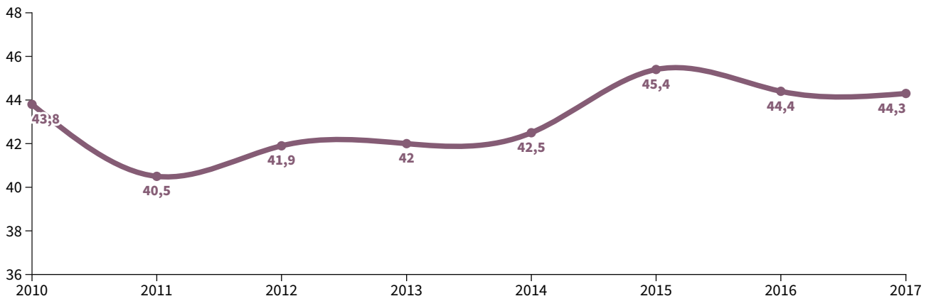
Şekil 163. PM2.5 Hava Kirliliği, Ortalama Yıllık Maruz Kalma Düzeyleri (Metreküp Başına Mikrogram, 2010-2017)
