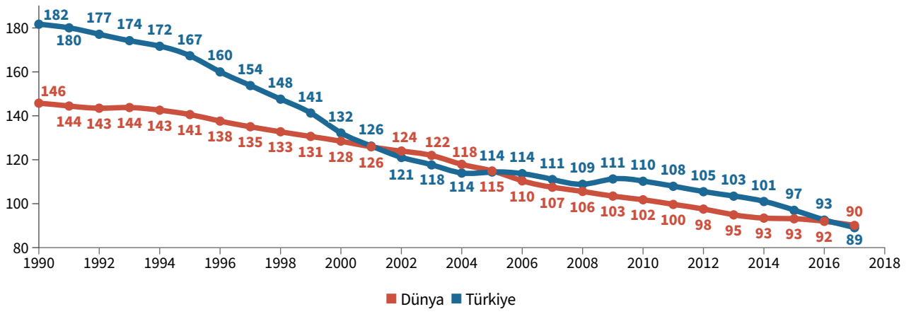
Şekil 191. Tütün Kullanımı Kaynaklı 100.000 Kişi Başına Ölüm (1990-2018)
